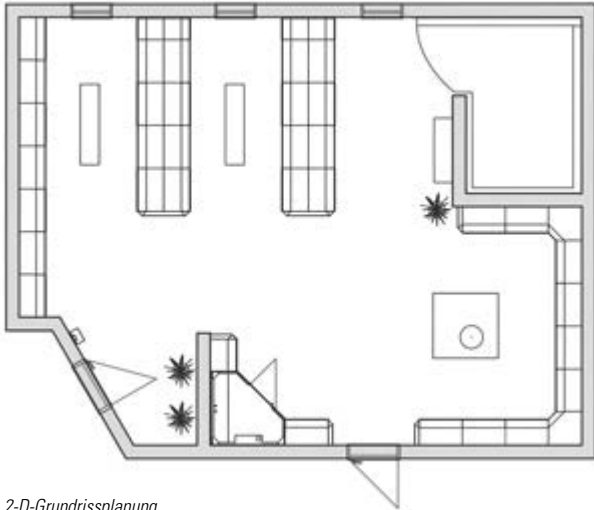
2-D-Grundrissplanung
